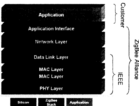
그림 1. ZigBee Protocol Stack Fig. 1. ZigBee Protocol Stack
