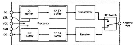
그림 4. Internal Data Flow Diagram Fig. 4. Internal Data Flow Diagram
