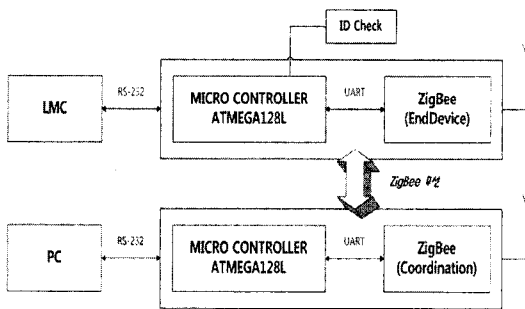
그림 5. 거리측정 시스템의 전체 블록도 Fig. 5. whole block diagram of distance measurement system
