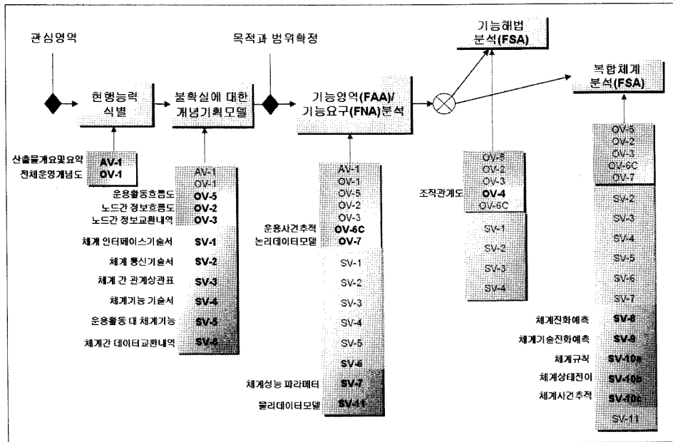
그림 3 JCIDS 소요도출/검토 단계별 아키텍처 활용
