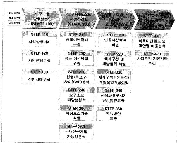
그림 5 아키텍처기반 선형연구수행절차
