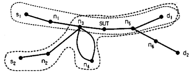
그림 2 통합 시험 형상 및 광역 시나리오
