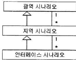
그림 1 상호운용성 시험 시나리오 계층 구조
