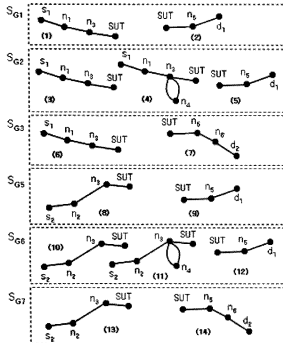
그림 4 광역시나리오로부터 도출된 지역시나리오 집합
