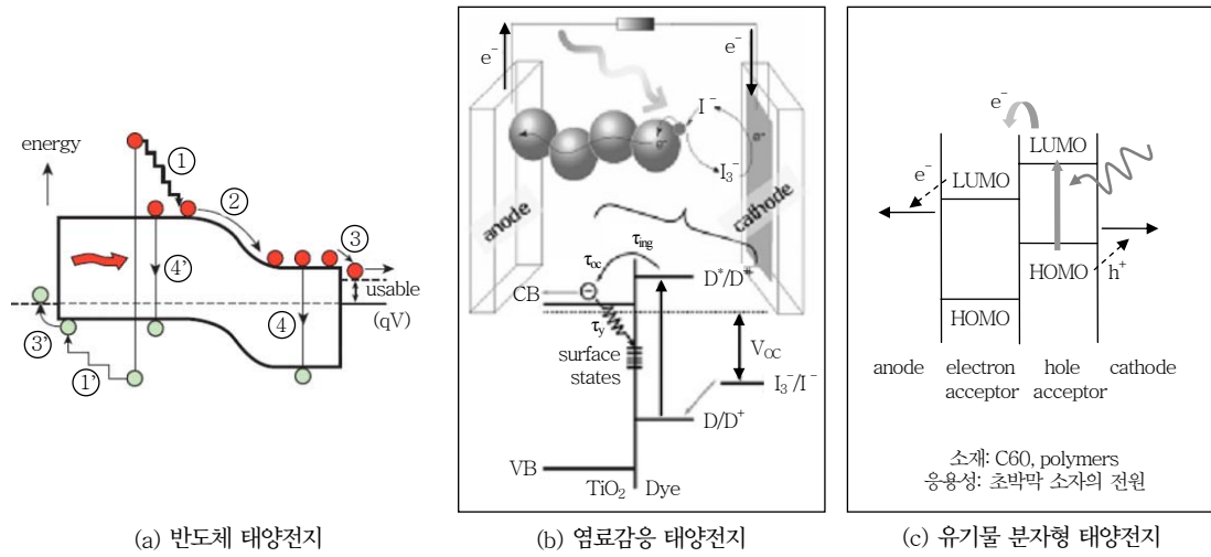
(그림 1) 다양한 태양전지의 광전 변환 원리
