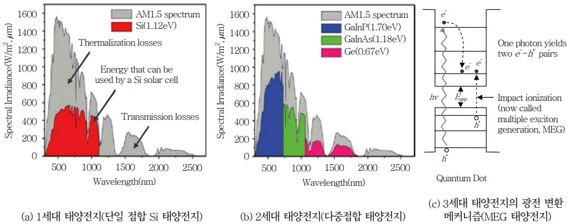
(그림 3) 태양전지 구조에 따른 광 흡수 대역
