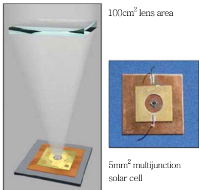
(그림 10) 집광형 태양전지
