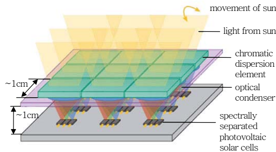
(그림 6) 초고효율 태양전지 배열 방식
