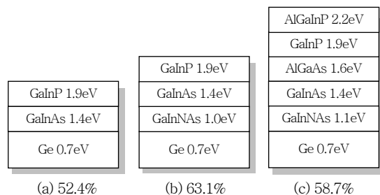
(그림 9) 다중 접합을 이용한 III-V 화합물 반도체 태양전지의 이론적 효율
