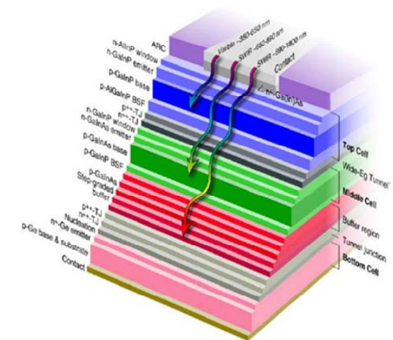
(그림 8) III-V 화합물 반도체를 이용한 GaInP/GaInAs/Ge 3중 접합 태양전지 구조
