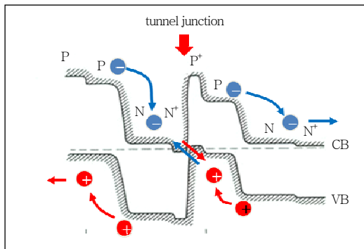
(그림 7) 터널정선 동작원리
