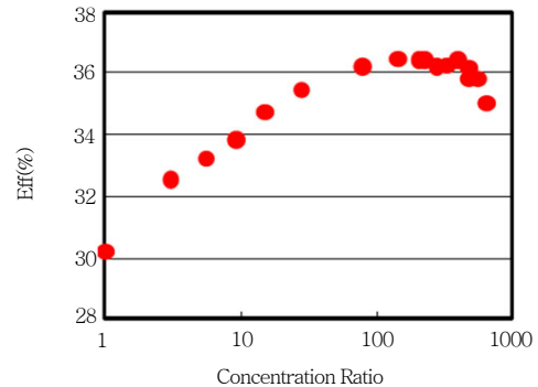
(그림 11) III-V 화합물 반도체의 집광 비율에 따른 효율 변화
