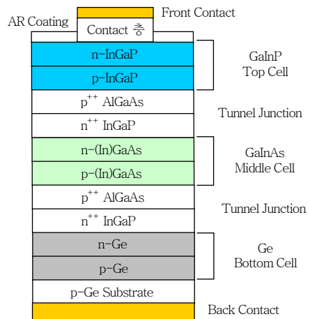
(그림 4) GaInP/GaInAs/Ge 3중 접합 태양전지 구조
