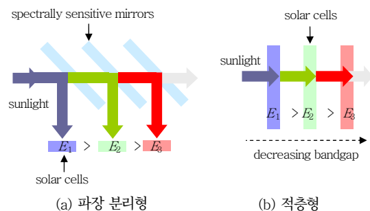
(그림 5) 다중 접합 태양전지 개념도
