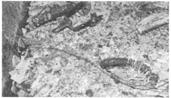
소형저장탱크 이충반밸브 접속구 용융이탈(액체라인)
