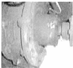
펌프와 삼방 밸브를 연결한 배관 파손
