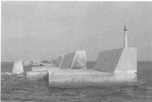
방파제의 피해 (1)
