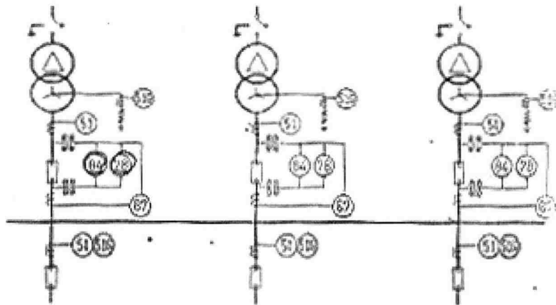
51 : 과전류계전기, 84 : 전압계전기, 78 : 위상계전기 51G : 지락과전류계전기, 67 : 전력방향계전기
