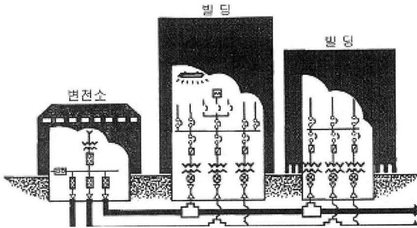
그림 3. Spot Network 배전선로
