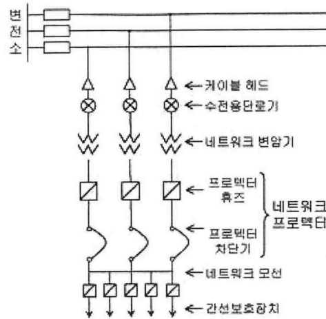
그림 1. Spot Network 배전방식
