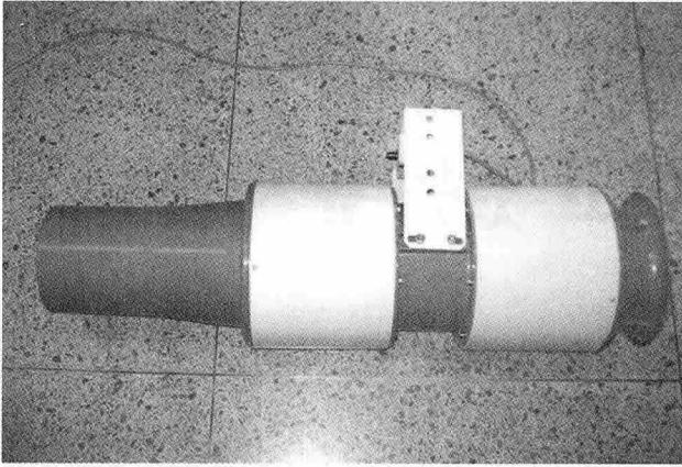
<그림 3> 새로운 증계팬(제트환기팬)
