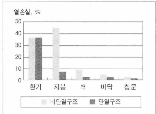
<그림 1> 축사에서 단열과 비단열의 열손실 비교, Scainsbury, 1995.
