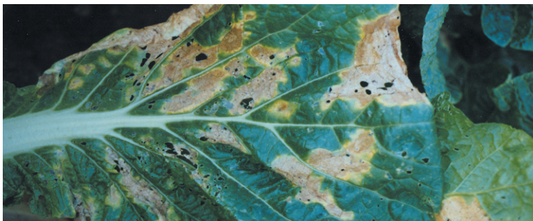
검은썩음병
