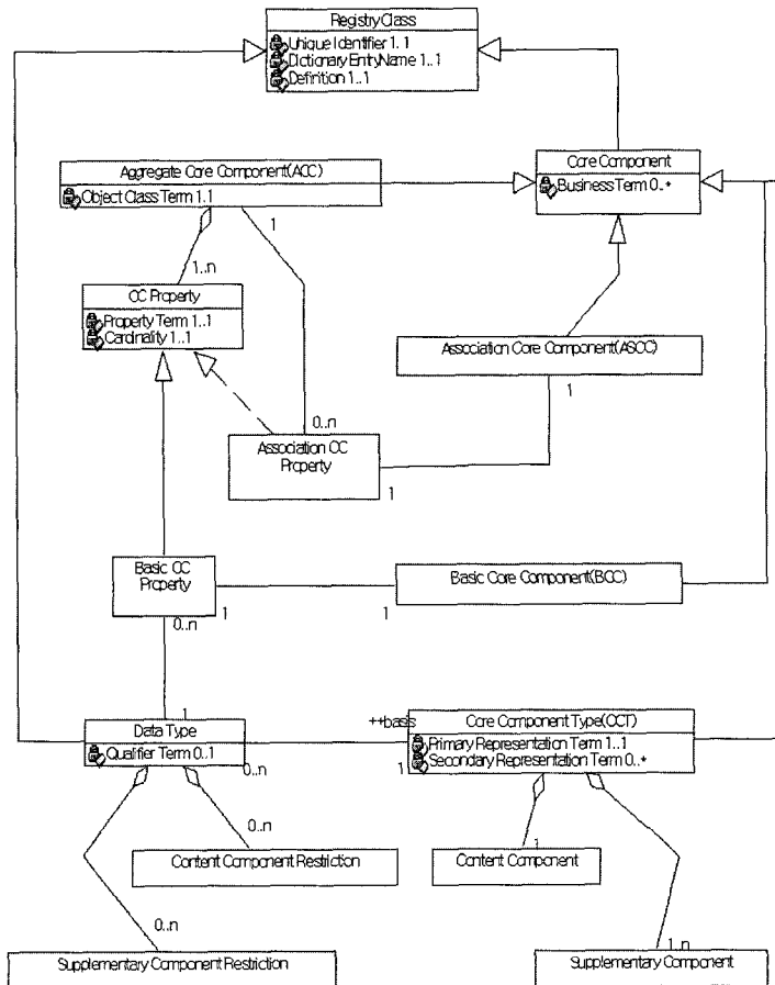
<그림 1> 코어 컴포넌트 구조
