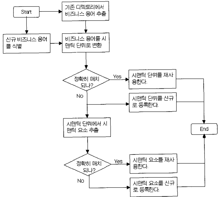
〈그림 3〉 시맨틱 라이브러리 개발 절차
