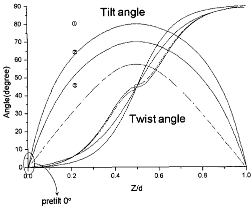
(a) 선각도 = 0°
