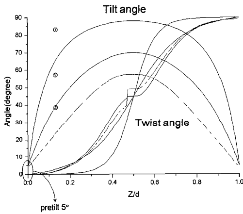
(b) 선각도 = 5°
