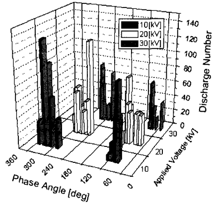
그림 2. \Phi -n 군집의 방전 횟수 분포 (구리).
