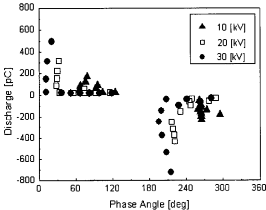
그림 5. \Phi -q 군집의 중심점 분포 (반도체재료). Fig. 5. Centroid distribution of \Phi -q cluster (semiconducting materials).
