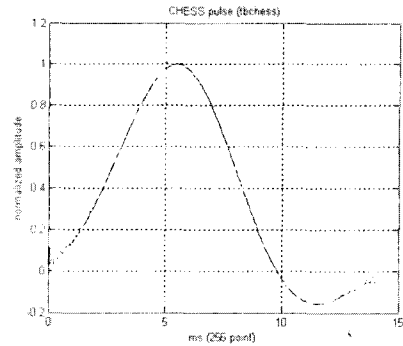
(그림 3) Design한 RF pulse
