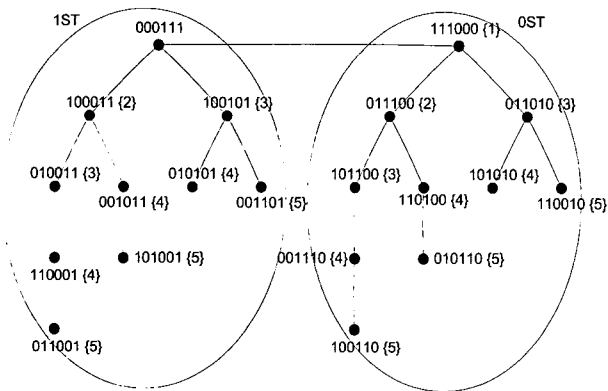
(그림 3) double rooted 스페닝 트리 DST(000111, 111000)
