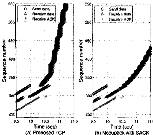
그림 6. 384 Kbps → 11Mbps 이동시 TCP-D 메커니즘의 시간(sec)당 보낼 수 있는 패킷의 양 비교
