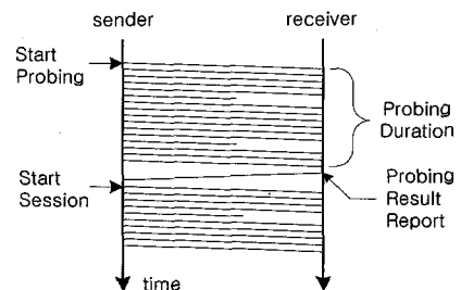
그림 1. 측정기반 수락제어 메커니즘 절차
