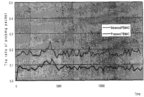
그림 9. 전체 전송 패킷에 대한 프루빙 패킷 비율
