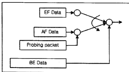
그림 6. 코어 노드에서의 스케줄링 방법
