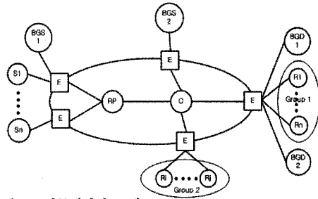
그림 7. 시뮬레이션 모델
