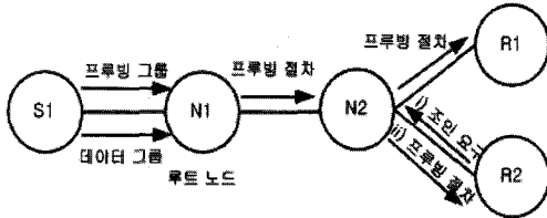
그림 4. Enhanced 프루빙 기반 멀티캐스팅 수락 제어 메커니즘
