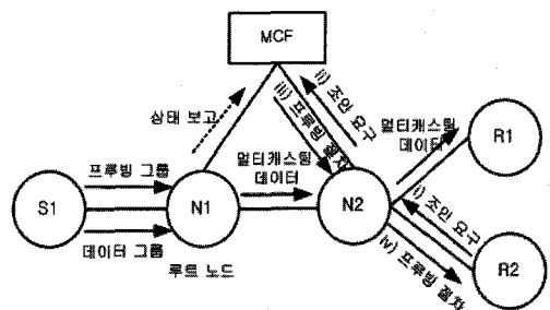
그림 5. 제안된 중앙 집중형 프루빙 기반 멀티캐스팅 수락 제어 메커니즘
