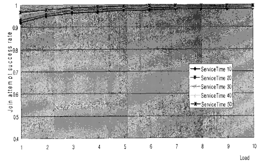
(a) 제안된 프루빙 기반 멀티캐스팅 수락제어 메커니즘
