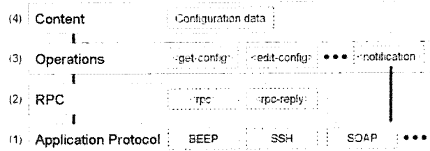
(그림 3) NETCONF 프로토콜의 계층 구조
