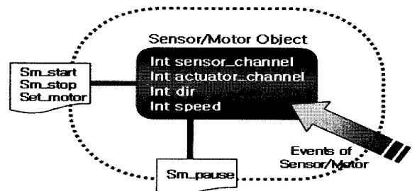
(그림 8) 센서/액추에이터 모듈의 구조
