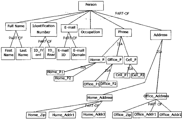
(그림 3) 개인 데이터 온톨로지
