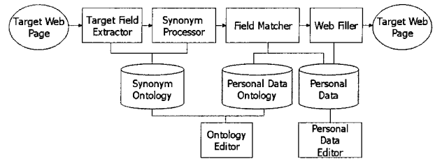
(그림 2) 제안된 시스템의 구조
