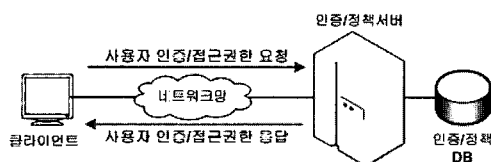
(그림 2) 일반적인 네트워크 시스템의 사용자 인증/접근제어
