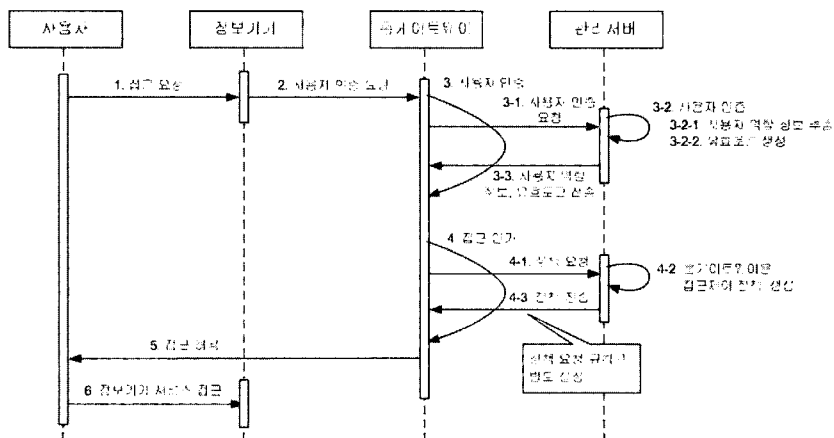
(그림 8) 홈 내부에서의 정보기기 서비스 접근 시퀀스
