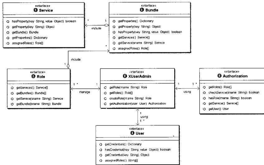
(그림 5) 사용자 인증 및 접근제어 서비스 인터페이스
