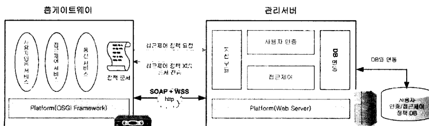
(그림 4) 원격관리서버 기반의 사용자 인증 및 접근제어 시스템 구성도
