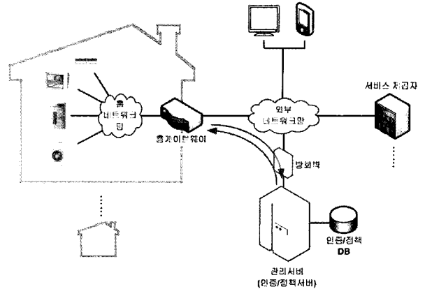
(그림 3) 원격관리서버 기반 사용자 인증/접근제어
