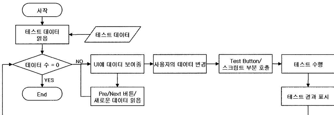
(그림 15) 클라이언트 페이지의 기능 테스트 드라이버 동작
