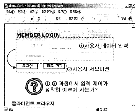
(그림 5) 클라이언트 측 페이지 입력 제어 기능 테스트 방법
