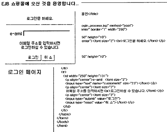
(그림 2) 정적 페이지
