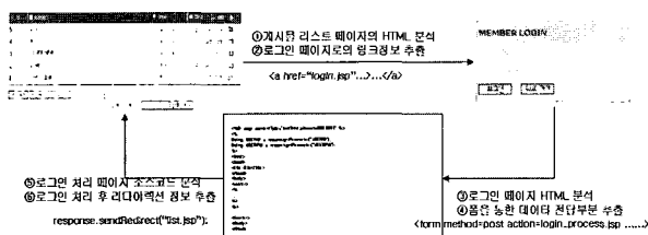
(그림 8) 정보 추출 과정
