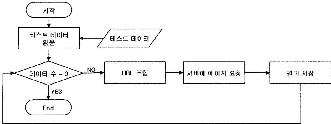
(그림 13) 서버 페이지의 기능 테스트 및 클라이언트 페이지의 UI 테스트를 위한 테스트 드라이버 동작
