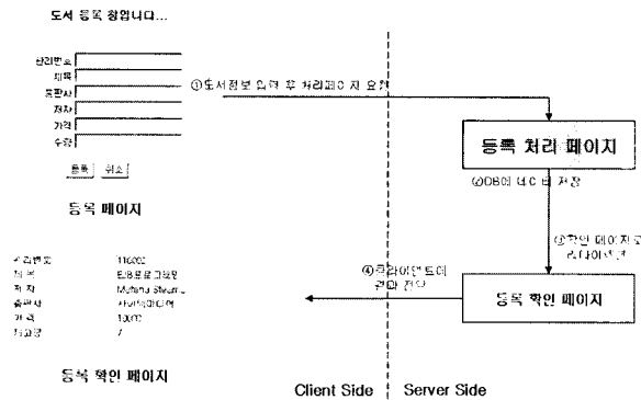
(그림 6) 서버 측 페이지
