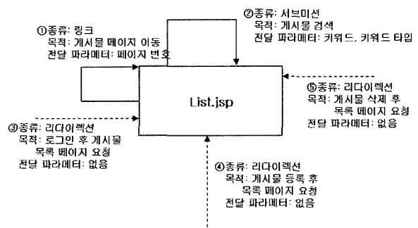
(그림 9) 게시물 목록 페이지의 요청
