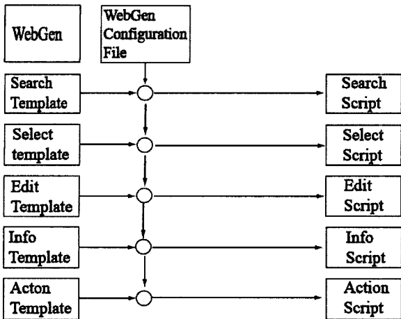
(그림 1) 템플릿 기반 WebGen
