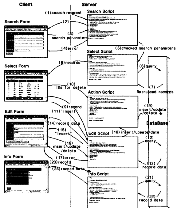
(그림 2) 생성된 웹 스크립트와 폼의 상호작용
