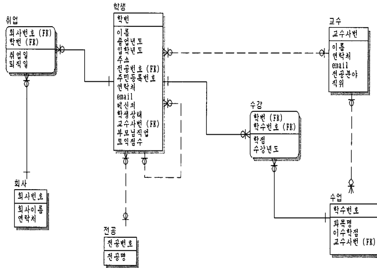
(그림 3) 정보공학대학 학생/졸업생 관리 응용의 ER 다이어그램
