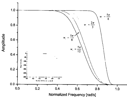
그림 5. L=2 일 때 w_c 에 따른 진폭응답 H_N(w)
