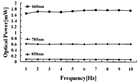
그림 6. 주파수에 따른 광 출력.
