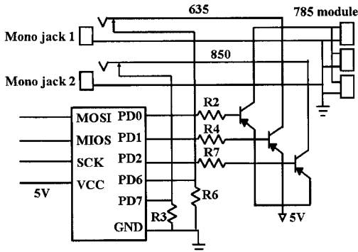
그림 3. 기기의 스위칭 회로. Fig. 3. Switching circuit of equipment.
