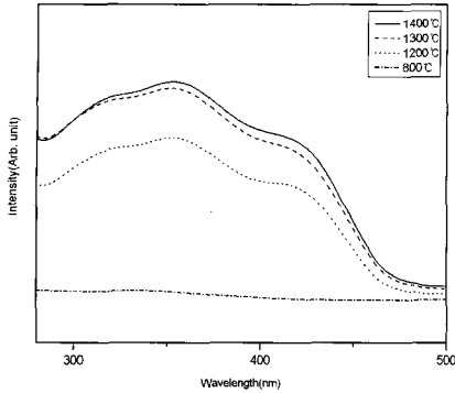
그림 8. 소성온도에 따른 SrAl 2 O 4 :Eu 2+ , Dy 3+ 형광체의 여기 스펙트럼.
