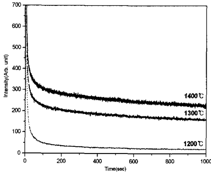
그림 10. 소성온도에 따른 SrAl 2 O 4 :Eu 2+ , Dy 3 형광체의 잔광 특성.
