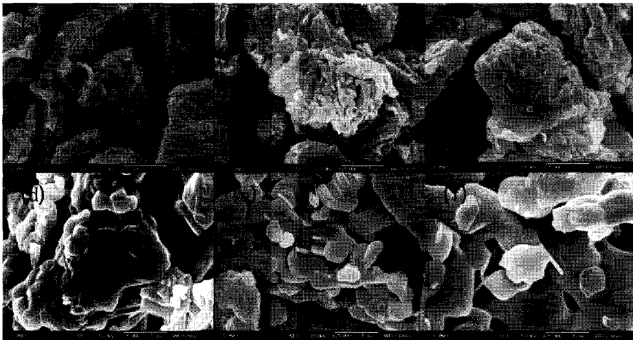
그림 7. 온도 변화에 따른 \text{SrAl}_2\text{O}_4:\text{Eu}^{2+}, \text{Dy}^{3+} 형광체의 SEM 사진: (a)900 °C, (b)1000 °C, (c)1100 °C, (d)1200 °C, (e)1300 °C, (f)1400 °C.
