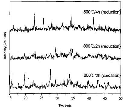
그림 5. 하소한 SrAl 2 O 4 :Eu 2+ , Dy 3+ 형광체의 X선 회절 패턴.
