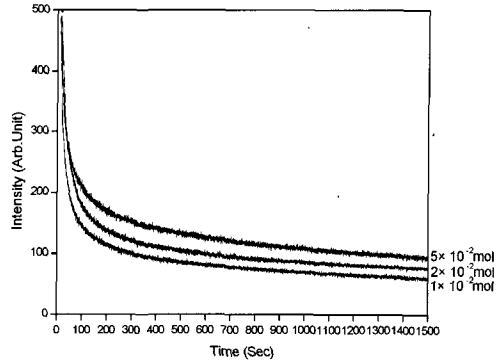
그림 11. 부활제 및 공부활제의 농도변화에 따른 SrAl 2 O 4 :Eu 2+ , Dy 3 형광체의 잔광 스펙트럼.
