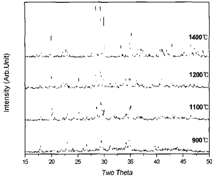
그림 6. 열처리 온도에 따른 \text{SrAl}_2\text{O}_4:\text{Eu}^{2+}, \text{Dy}^{3+} 형광체의 X 선 회절 패턴.
