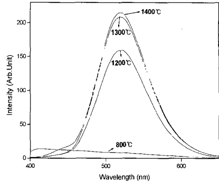
그림 9. 소성온도에 따른 SrAl 2 O 4 :Eu 2+ , Dy 3+ 형광체의 발광 스펙트럼.
