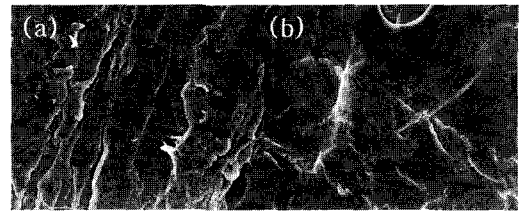
그림 2. 결정성 셀룰로오스와 함침된 고분자 전구체의 Microfibril 구조.
