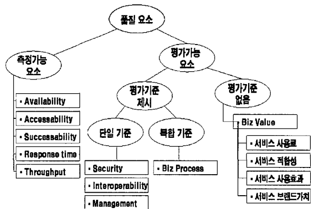
(그림 7) 품질요소 구분
