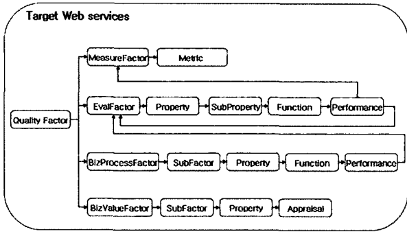
(그림 8) 품질항목 데이터 구조
