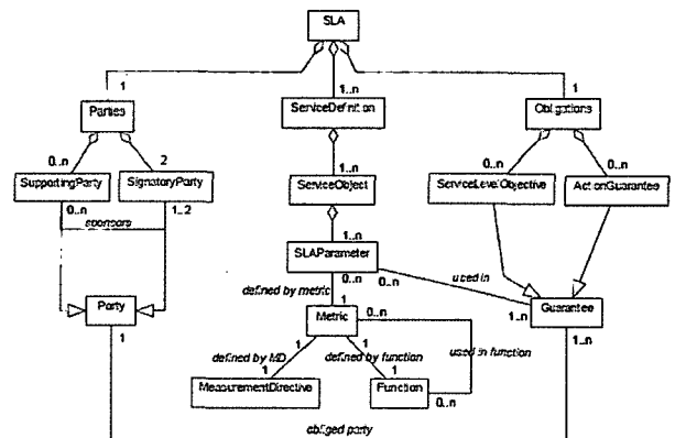
(그림 2) WSLA 개념 개요
