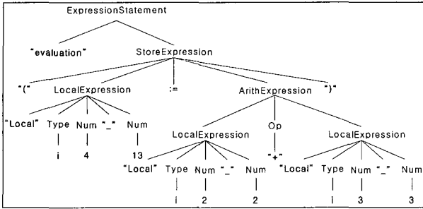
(그림 6) <ExpressionStatement> 구조
