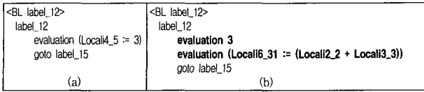
(그림 8) 표현식 추가전과 후의 모습
