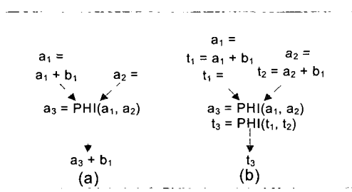
(그림 1) 부분 중복 표현식 제거
