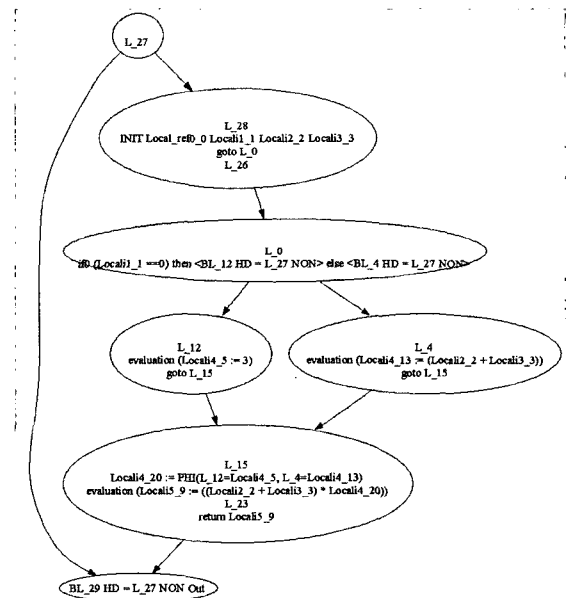
(그림 12) SSA Form
