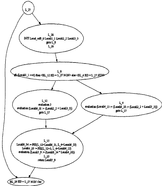
(그림 13) 부분 중복 제거 후
