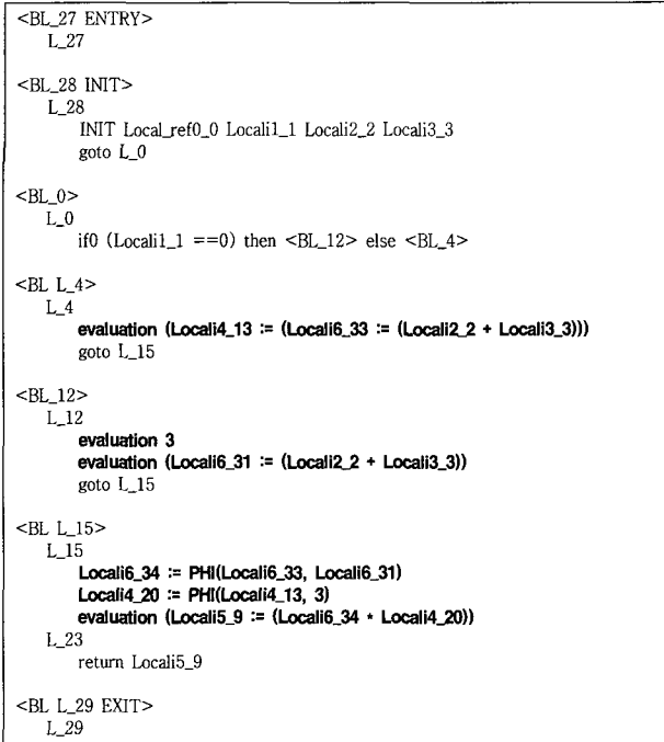
(그림 9) PRE 적용 후 SSA Form 형태의 CFG
