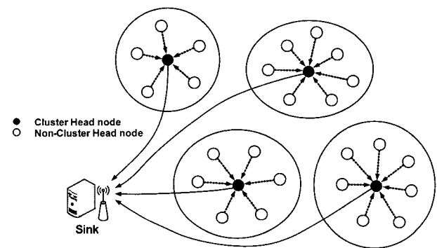
(그림 1) 클러스터 기반의 라우팅 프로토콜 구조
