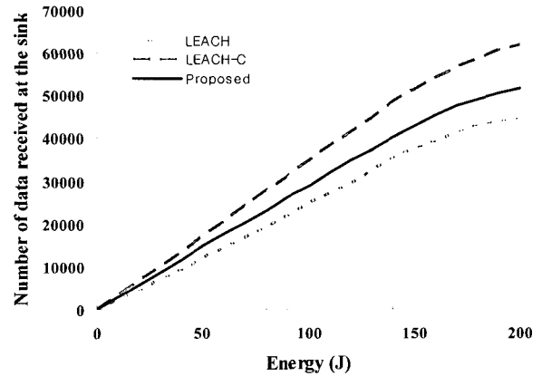
(그림 5) 에너지 소비량에 따른 데이터 전송량
