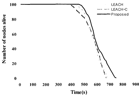
(그림 4) 시간에 따른 잔여 에너지가 남아있는(alive) 노드의 수
