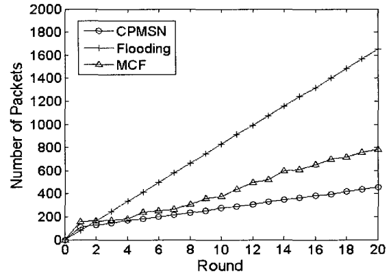
(그림 10) 누적 트래픽 오버헤드
