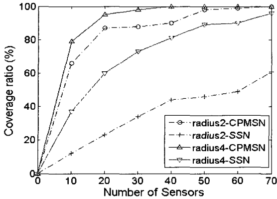
(그림 7) 센서의 개수와 센싱 반경에 따른 네트워크 커버리지 (%)
