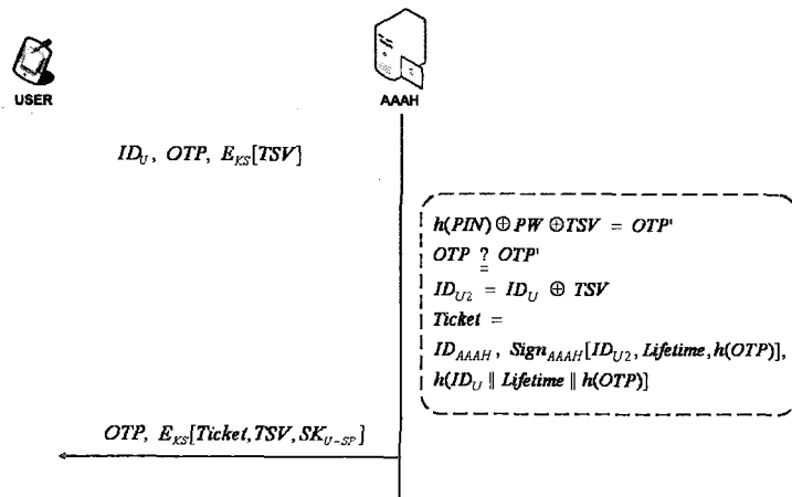
(그림 2) 티켓 및 인증 요청 단계
