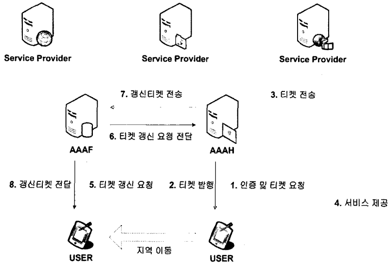
(그림 1) 제안 방식 전체 흐름도
