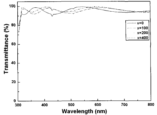
그림 10. 첨가량 변화에 따른 MgO 박막의 가시광영역에서의 투과율.
