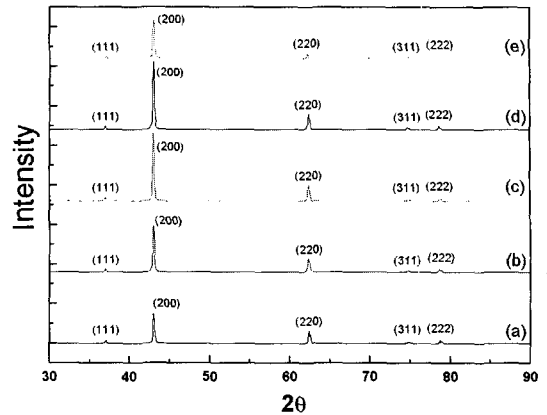
그림 4. 1700 °C에서 5시간 소결한 보호막의 Gd 2 O 3 첨가량 변화(x = 0, 100, 200, 300, 400)에 따른 X선 회절 패턴.
