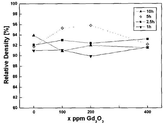
그림 2. Dopant 첨가량과 소결시간에 대한 상대 밀도. Fig. 2. Relative density of MgO + x ppm Gd 2 O 3 as a function of Gd 2 O 3 content and sintering time(1, 2.5, 5, 10 hrs).
