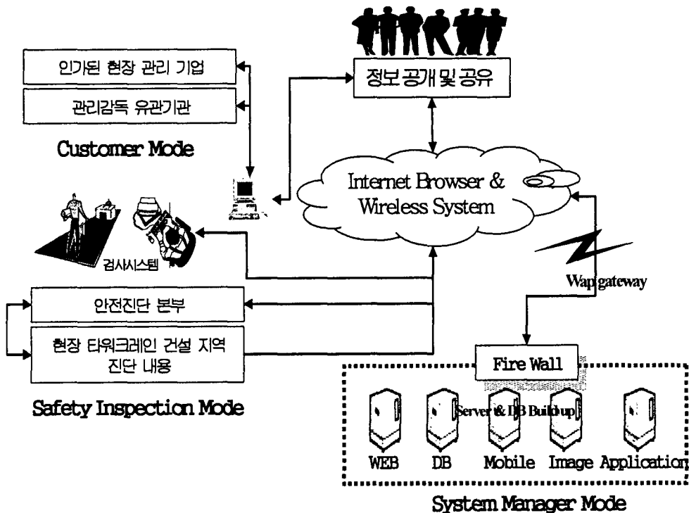
<그림 3> 타워크레인 관리시스템 구성도
