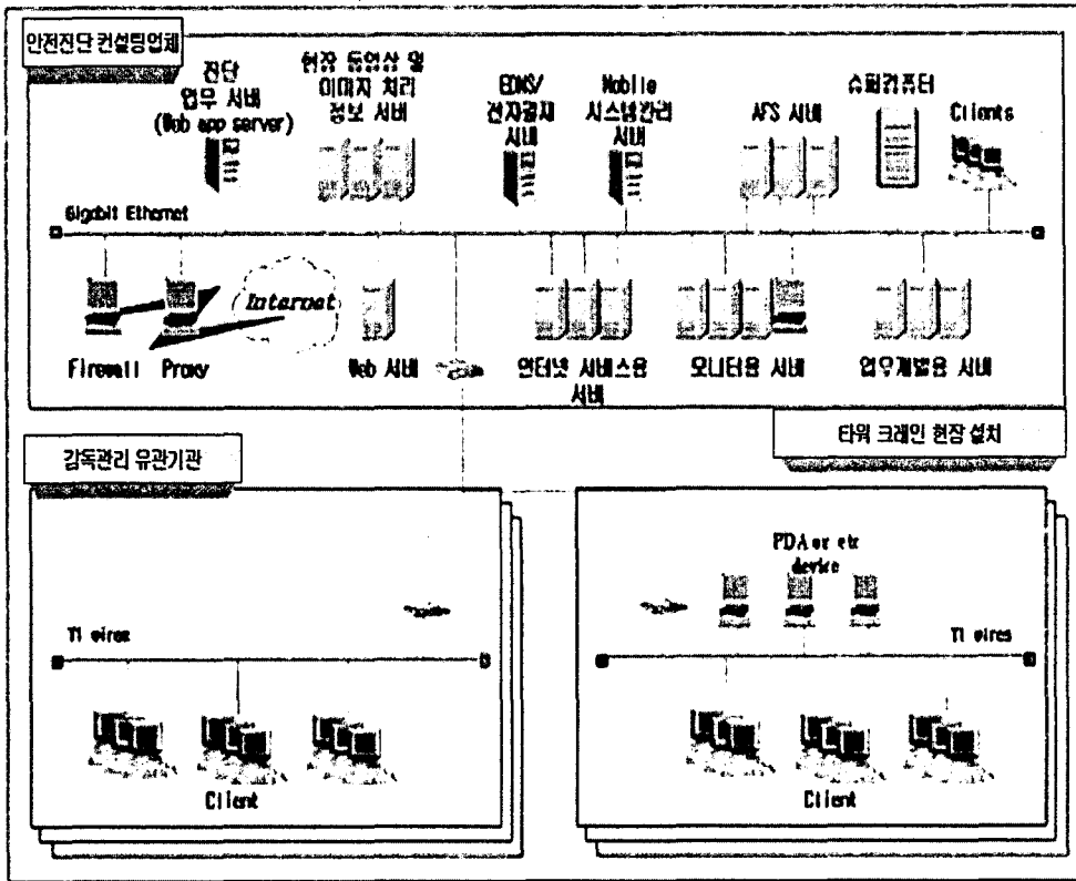
<그림 4> 타워크레인 진단시스템 Infra Architecture
