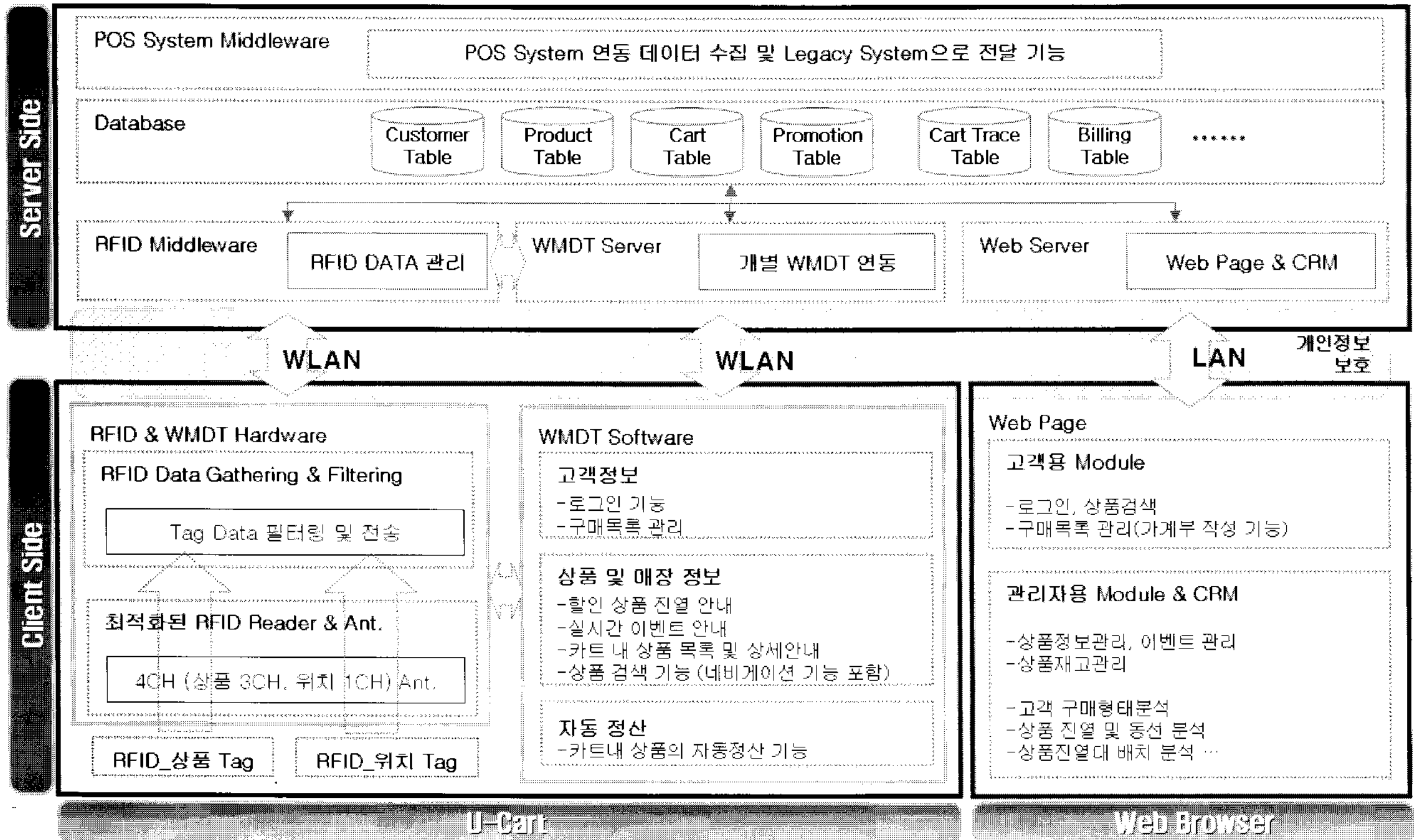
<그림 3> RFID 기반의 이동형 u-POS 시스템의 S/W 구성도
