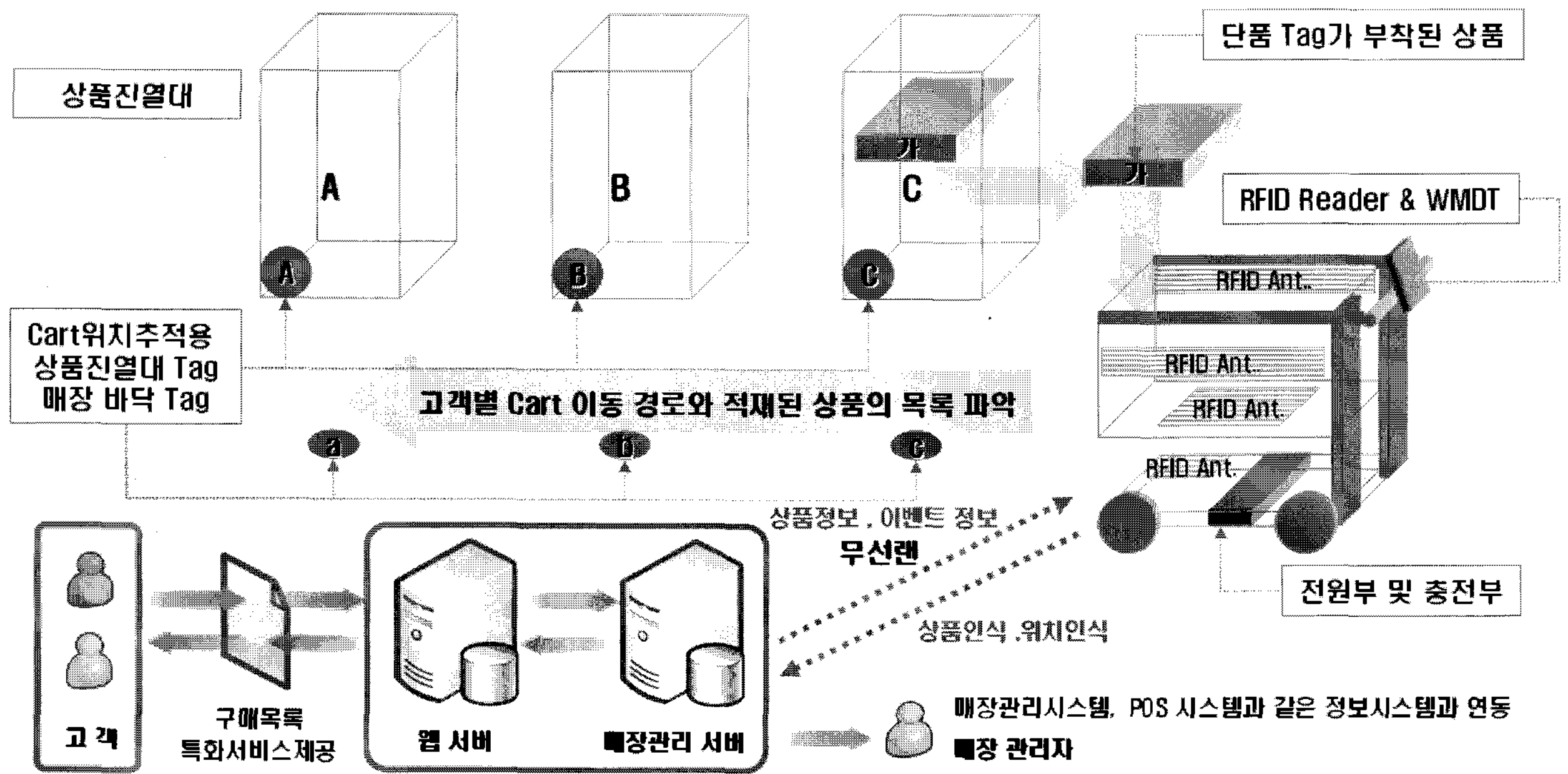
<그림 1> RFID 기반의 이동형 u-POS 시스템의 H/W 구성도
