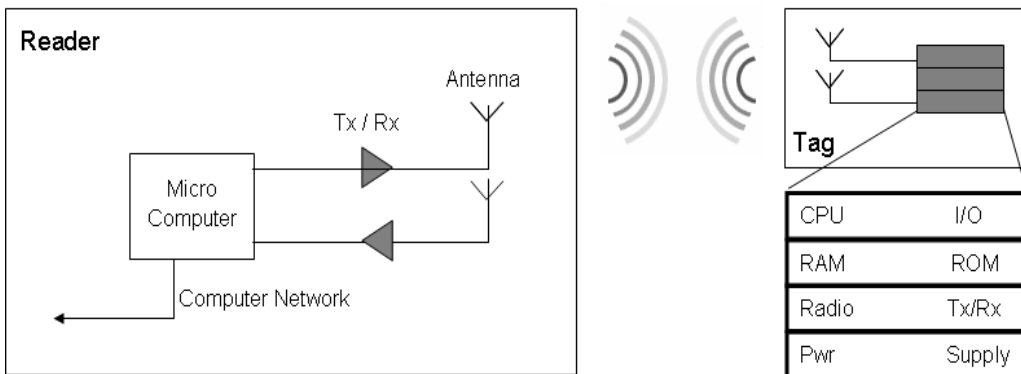
그림 1. RFID 시스템 구성도
