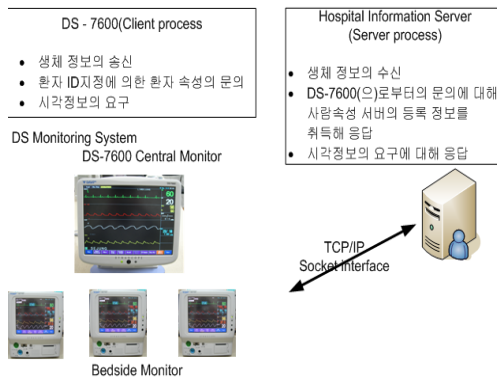
그림 1. 생체정보 전송 시스템 Fig. 1 Vital sign information transfer system
