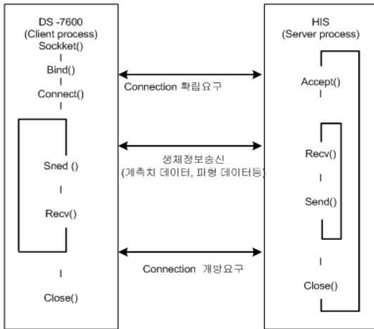
그림 3. 생체정보의 통신 순서 Fig. 3 Vital sign socket procedure
