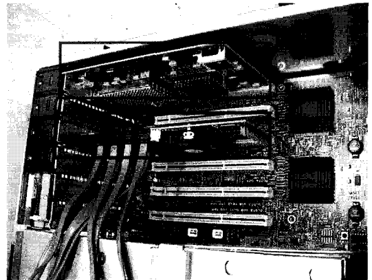
그림 4. AMD 시스템(10 기가급 네트워크 장치(상단), 레이드 디스크 제어장치(하단))
