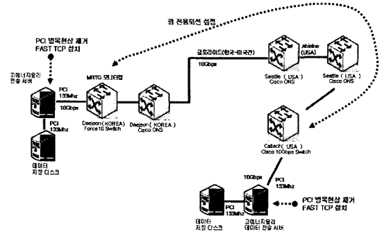
그림 6. 테스트베드 구성도
