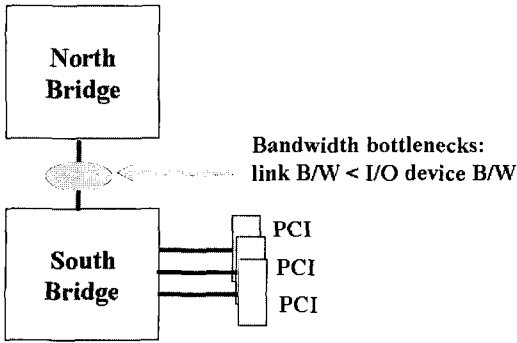
그림 2. PCI 병목현상 ([5]에서 그림 인용)
