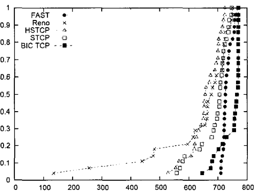
그림 5. 여러 TCP 들의 성능 비교 (X축: 전송률, Y축: CDF(Cumulative Distribution Function), 1 Gbps 대역의 네트워크에서 실험, [6]에서 그림 인용)
