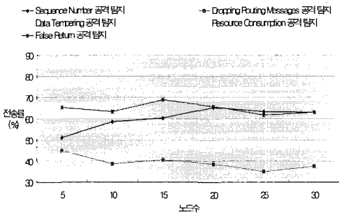
그림 11. 제한한 공격 탐지 시 전송률 (참여 노드수 변경)
