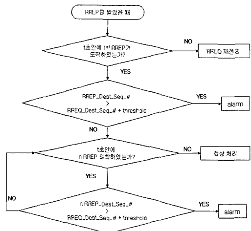
그림 2. Sequence Number 공격 탐지 순서도 (소스노드가 RREP 메시지를 받았을 때)
