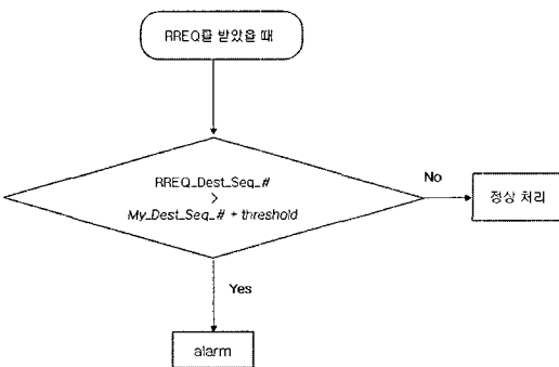
그림 4. Sequence Number 공격 탐지 순서도 (목적지노드가 RREQ 메시지를 받았을 때)
