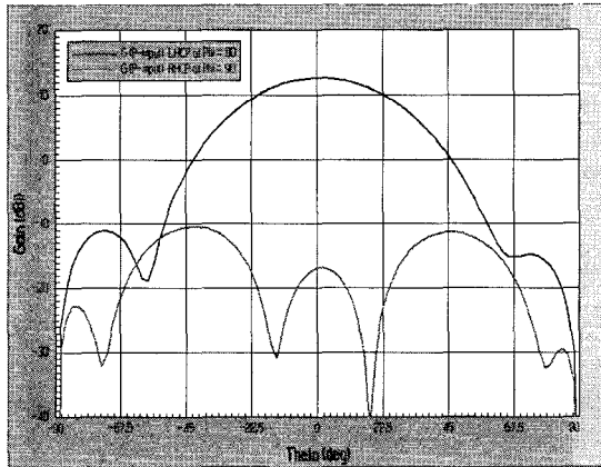
(b) H-plane
