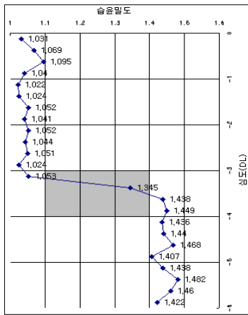
FIGURE 10. J1지점 습윤밀도
