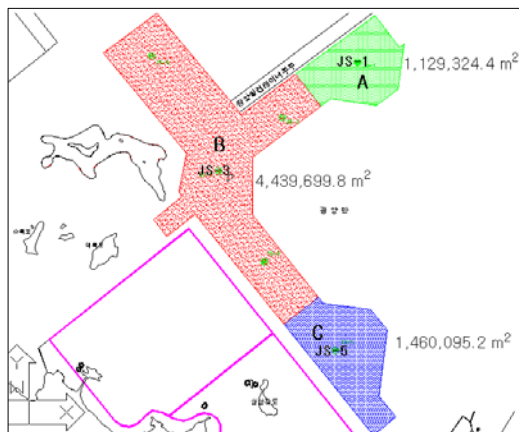
FIGURE 14. 지점별 준설예정구역 면적도
