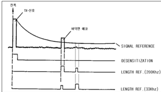
FIGURE 7. 주파수별 진폭의 변화
