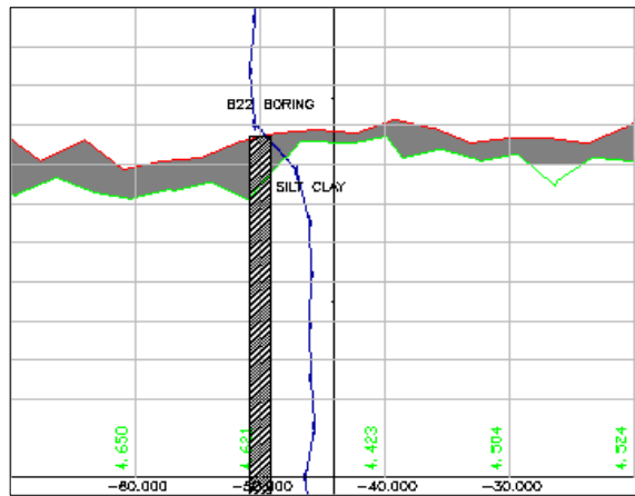
FIGURE 11. JS-1지점 부니층 분석도
