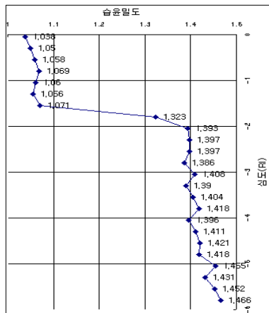
FIGURE 12. JS-5지점 습윤밀도
