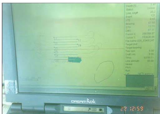
FIGURE 5. 선박의 항적유도(JS-3지점)
