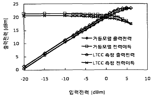
그림 5. 제작한 전력증폭기의 1-tone 측정결과와 거동모델 1-tone 시뮬레이션 결과 비교
