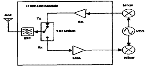
그림 1. IEEE 802.11a 시스템의 Front-End Module
