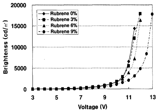
그림 3. Rubrene이 첨가된 OLED 소자의 인가전압에 대한 발광휘도. Fig. 3. Brightness versus applied voltage of rubrene doped OLED devices.
