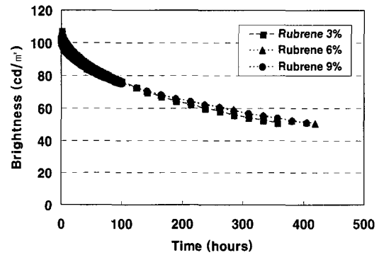
그림 7. Rubrene이 첨가된 OLED 소자의 rubrene 첨가량에 대한 발광수명.
