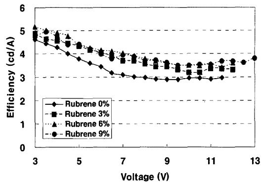
그림 4. Rubrene이 첨가된 OLED 소자의 인가전압에 대한 전류 발광효율. Fig. 4. Current efficiency versus applied voltage of rubrene doped OLED devices.
