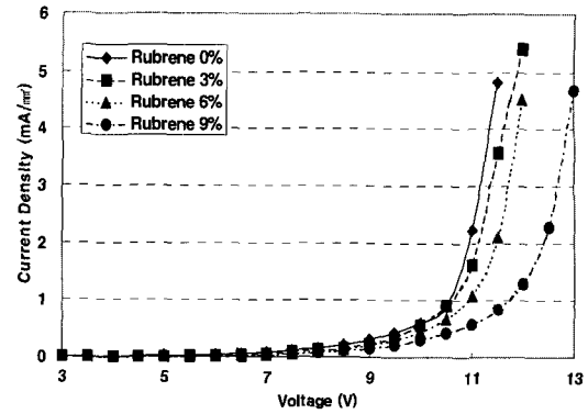
그림 2. Rubrene이 첨가된 OLED 소자의 인가전압에 대한 전류밀도.
