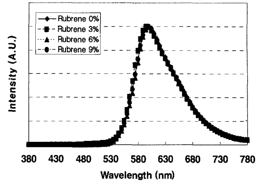
그림 6. Rubrene이 첨가된 OLED 소자의 rubrene 첨가량에 대한 발광스펙트럼.
