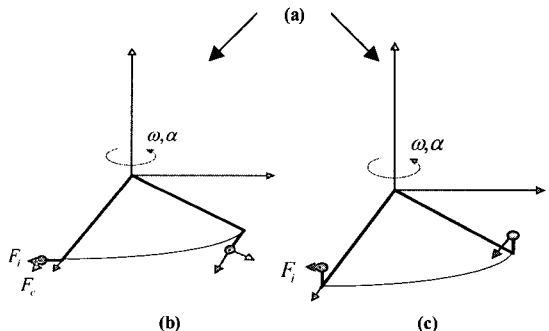
Fig. 11 (a) 3차원 스윙 운동, (b) 굽힘 운동 모델링, (c) 비틀림 운동 모델링.
