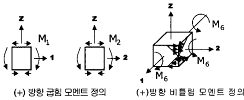
Fig. 3 모멘트 요소의 (+) 방향 정의.
