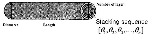
Fig. 2 샤프트의 정적특성 분석을 위한 파라미터.
