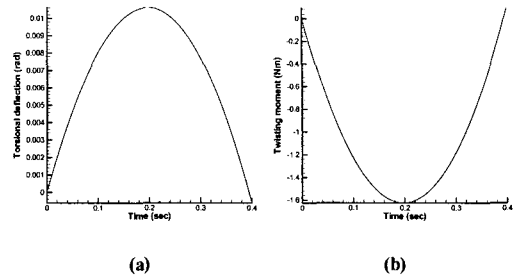
Fig. 14 (a) 헤드부근 샤프트 끝단의 비틀림 변위, (b) 그립부근 샤프트 끝단의 비틀림 모멘트.
