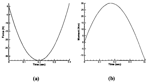
Fig. 13 (a) 그립부근 샤프트 끝단의 힘 (b) 그립부근 샤프트 끝단의 굽힘 모멘트.
