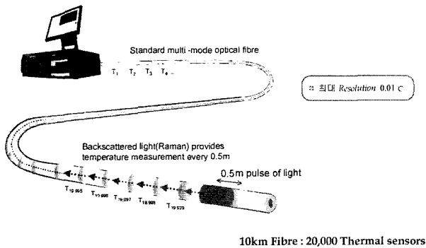
그림 4. 광섬유센서 케이블을 이용한 DTS 온도 측정기법의 원리 (Sensonet, sentinel DTS product research)
