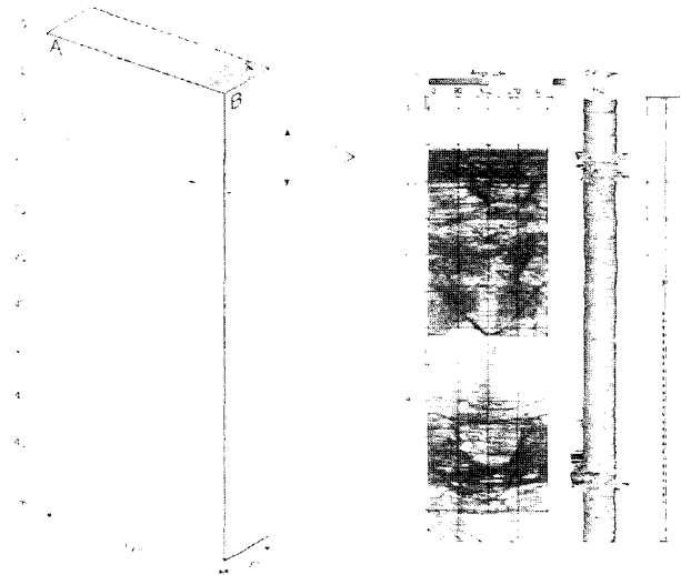
그림 14. 그라우팅 시험구간의 4개 시추공(MDB-5, GBH-1, GBH-2 및 GBH-3)에 대한 절리층세 밀도의 입체영상, 온도 모니터링공에 대한 텔레뷰어 이미지와 온도센서 배설 케이블의 놓인 위치
