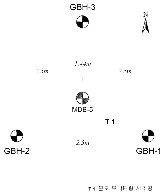
그림 13. 그라우팅 시험구간에서 온도센서 배열 케이블 설치를 위한 온도 모니터링 시추공(T1)의 위치
