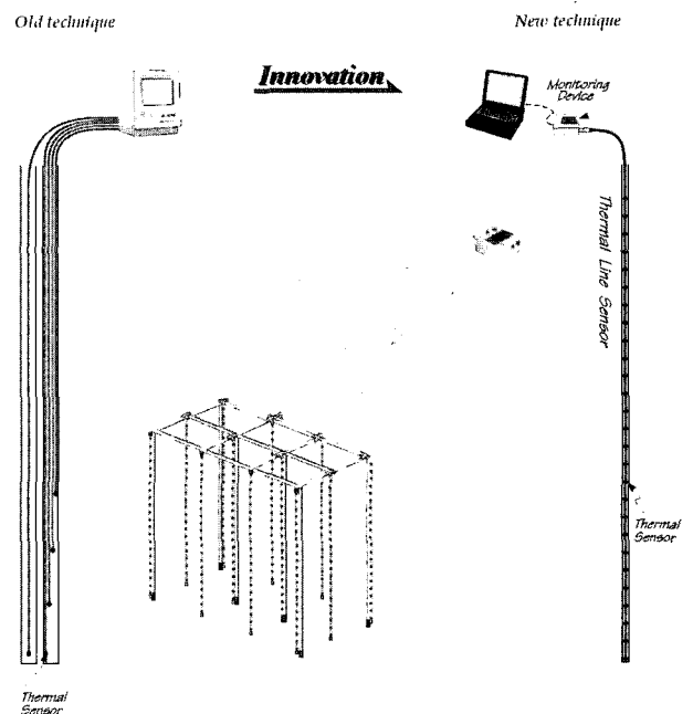
그림 1. 온도센서 배열 케이블을 이용한 온도모니터링 시스템
