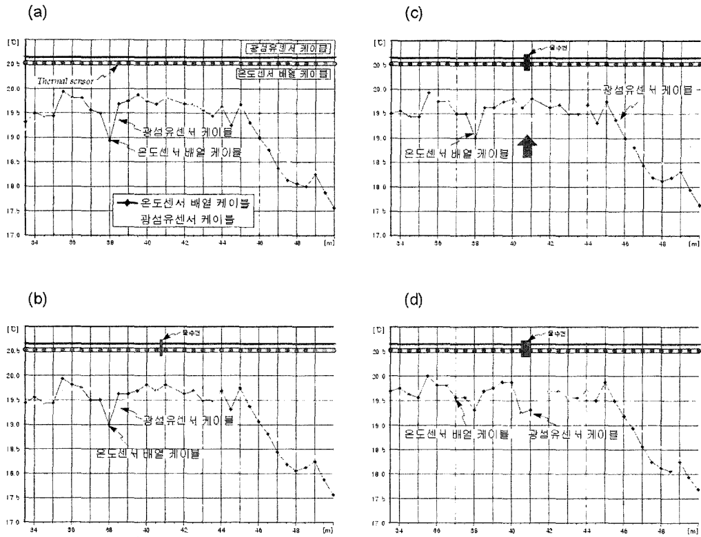
그림 9. 두 개 케이블 구간
