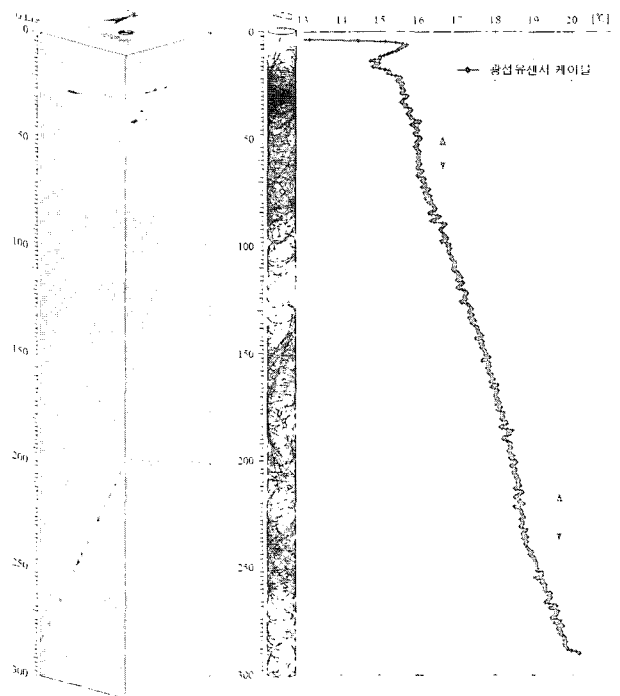
그림 16. 한국지질자원연구원 실험시추공에서 얻은 절리구조 3차원 입체 영상, 3D-Log 및 광섬유센서 케이블에 의한 온도 측정 결과의 상호대조
