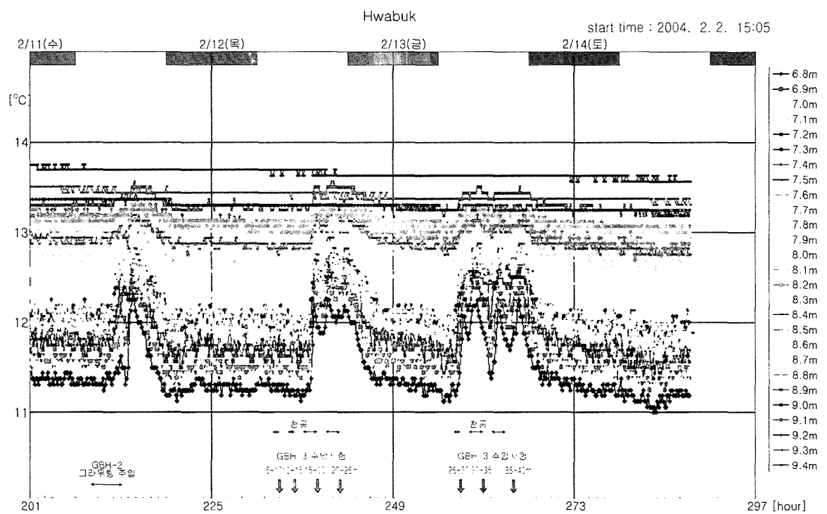
그림 15. 그라우팅 시험구간에서 온도센서 배설 케이블을 이용한 온도모니터링 결과
