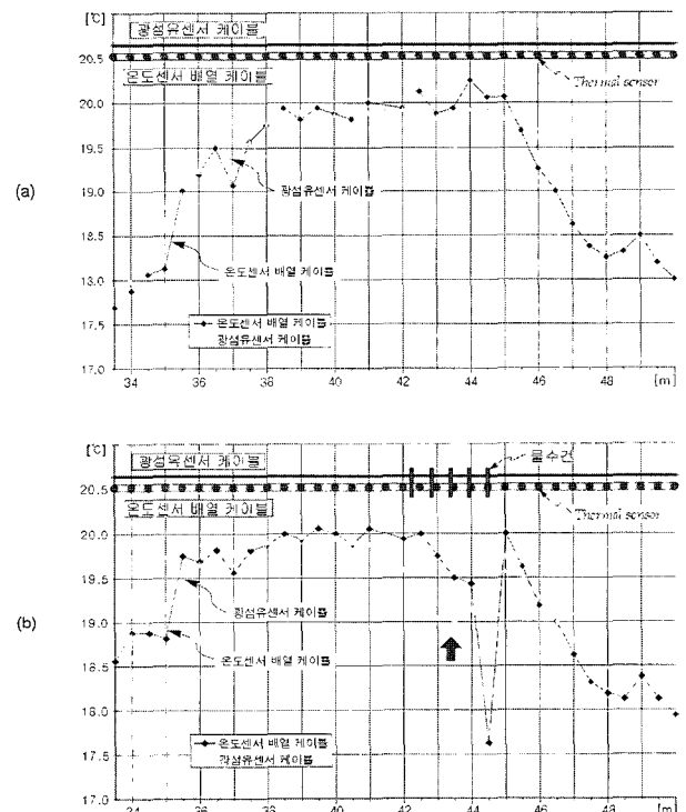
그림 6. 온도센서 배열 케이블과 광섬유센서 케이블의 측정 결과 비교 (a) 상온에서의 측정 결과 (b) 42.25m~44.50m 구간에 5개의 찬 물수건으로 온도변화를 준 후 측정 결과
