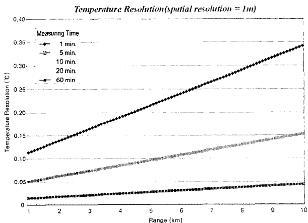
그림 5. 거리 및 측정시간에 따른 DTS의 온도분해능(Sensonet, sentinel DTS product research)
