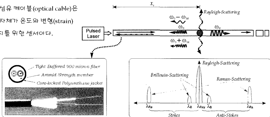
그림 3. 광섬유센서 이용기술의 근본원리
