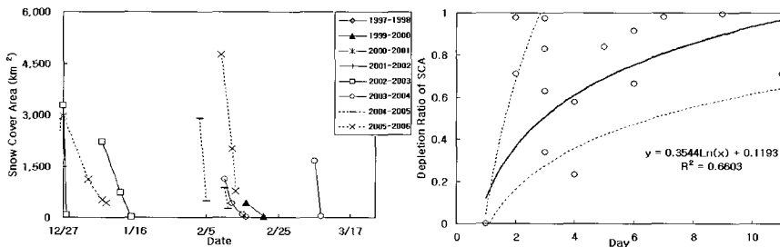
(e) 섬진강유역
