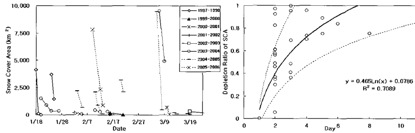
(b) 낙동강유역
