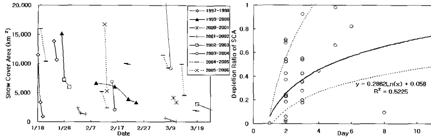
(a) 한강유역
