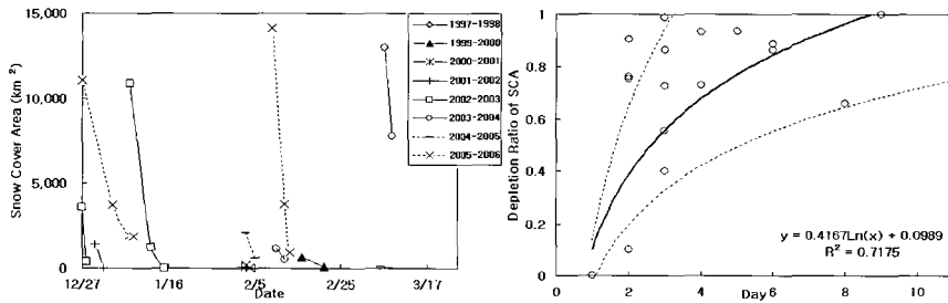
(c) 금강유역
