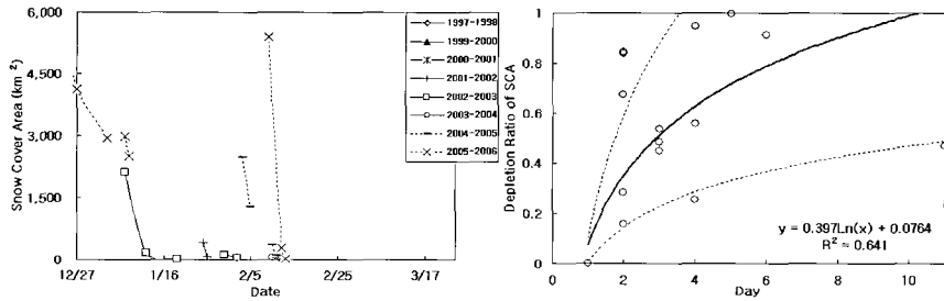
(d) 영산강유역
