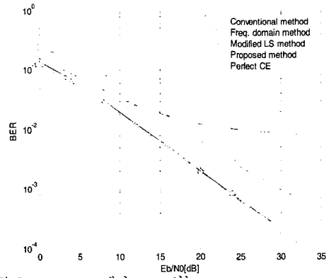
그림 3. f_d = 40 Hz에서 BER 성능 Fig. 3. BER performance at f_d = 40 Hz
