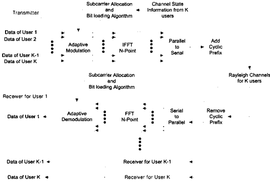
그림 1. 다중 사용자 OFDM 시스템 구조
