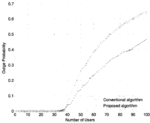
그림 4. 알고리즘 간의 outage 확률 비교
