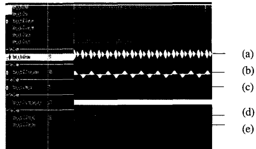
그림 5. 수신부 시뮬레이션 결과((a)수신신호, (b)정합기 출력 신호, (c)필터 출력 신호, (d)평균치, (e)검출 신호) Fig. 5 Receiver Simulation Result ((a)received signal, (b)matched filter output signal, (c)filter output signal, (d)average value, (e)detection signal)
