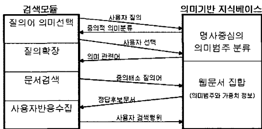
그림 1. 의미정보에 기반한 정보검색 흐름
