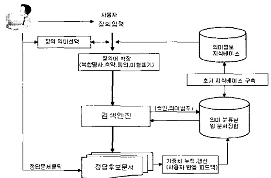
그림 4. 의미정보에 기반한 검색시스템의 구성
