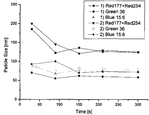
그림 6. 밀링 시간에 따른 밀베이스 분산도. Fig. 6. Time dependence of millbase dispersity.
