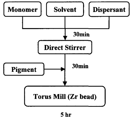
그림 1. 밀베이스의 제조 단계.
