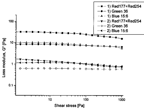
그림 8. 전단 응력에 따른 조성비 1), 2)의 RGB 밀베이스 손실탄성율.
