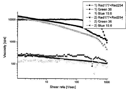
그림 7. 전단 속도에 따른 조성비 1), 2)의 RGB 밀베이스 점도. Fig. 7. Shear dependent viscosity of RGB millbase for fomulation 1), 2). (Retention time : 150s, Rate range : 0.1~1,000 1/s).
