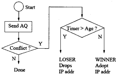
(b) RADA 주소 충돌 해결. (b) RADA Address Collision Resolution
