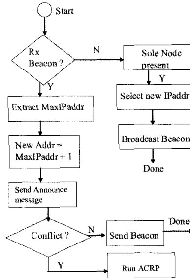
(a) LiA 주소 요청 (a) LiA Address Request
